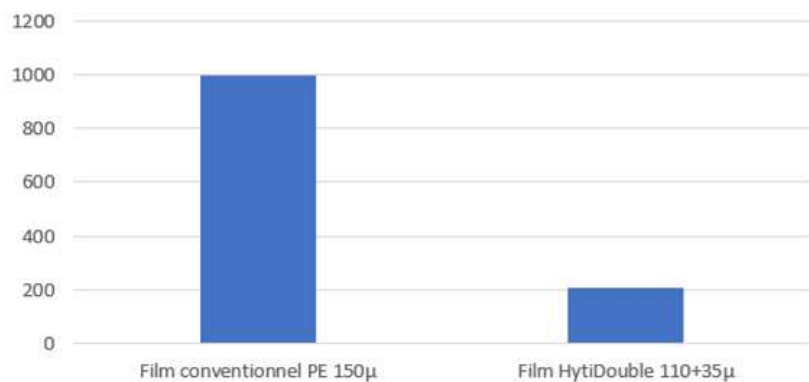
Comparatif de Porosité à l'oxygène en cm 3 /m 2 en 24 h
